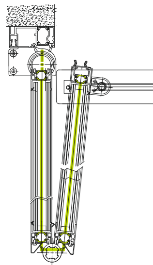
Thermal separation
